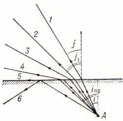
Рис. 1. Полное внутреннее отражение (луч 6) происходит при угле падения света на поверхность оптически менее плотной среды, превышающего критический угол i_{пр} , для к-рого угол преломления j составляет 90^\circ (луч 5). А — источник света. Показатель преломления нижней среды больше показателя преломления верхней.
